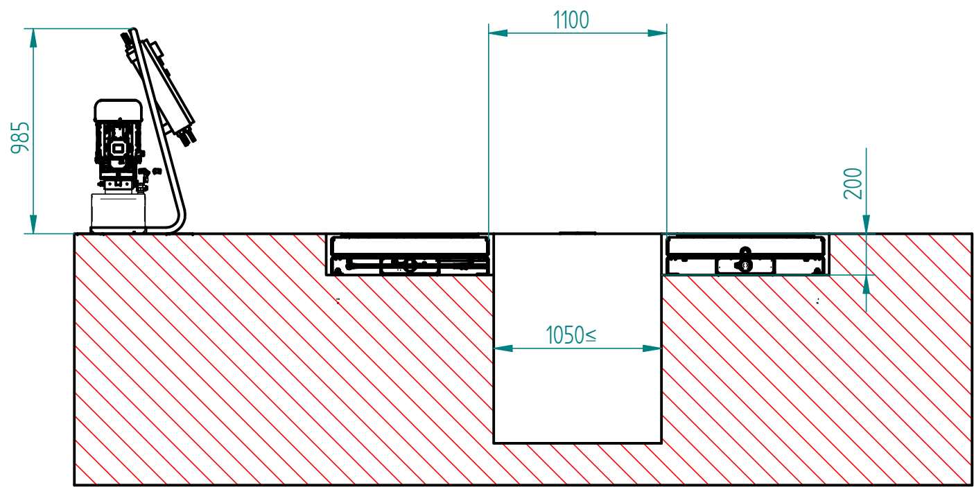
Sezione/Section A-A
