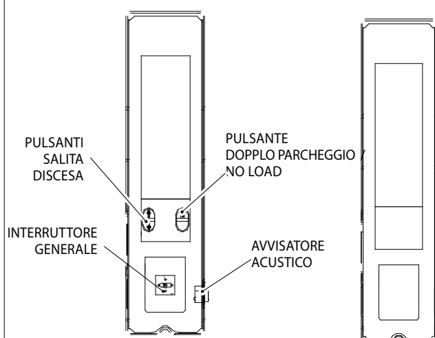
Codice impianto elettrico 049803210 049803220
