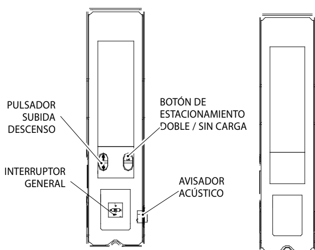
Código sistema eléctrico 049803210 049803220
