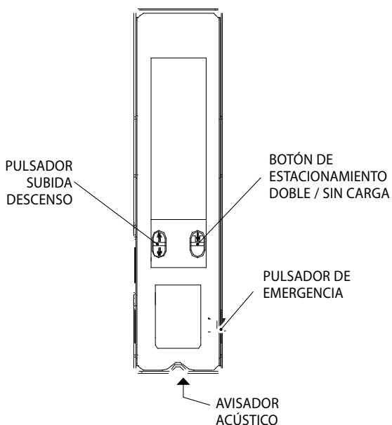
Código sistema eléctrico 049803240
