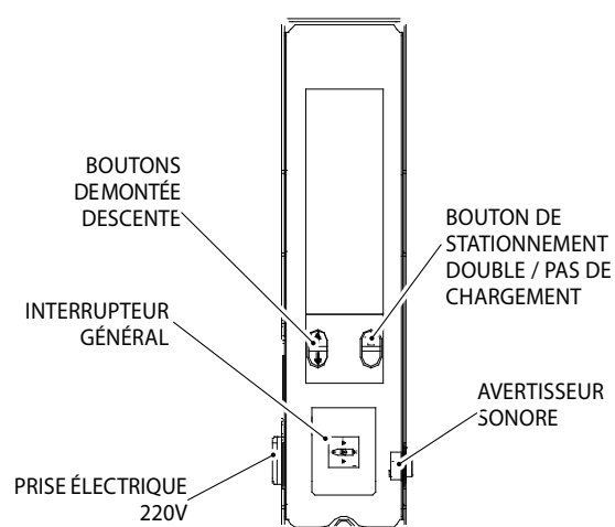
Code de l'installation électrique 049803230
