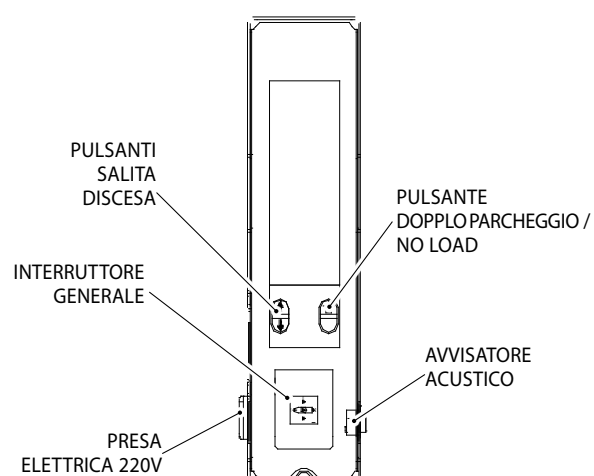
Codice impianto elettrico 049803230
