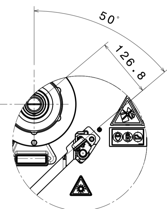
LASER SPOT Dettaglio B Scala: 1:5
